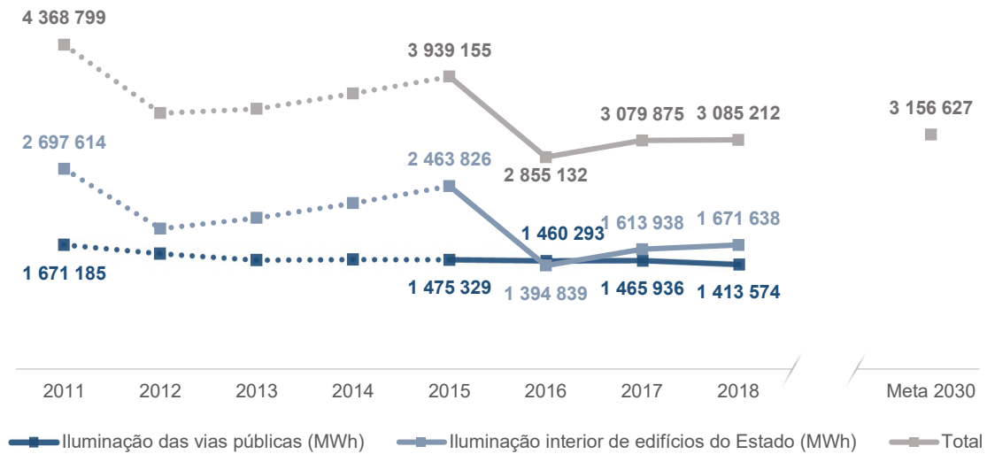
Consumo de energia elétrica para iluminação das vias públicas e iluminação interior de edifícios do Estado (kWh) - Portugal
