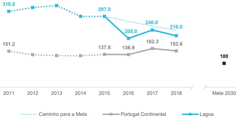
Perdas reais de água [m 3 /(km.dia)] ou [l/(ramal.dia)]
